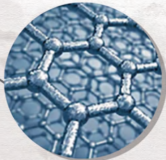
石墨烯
